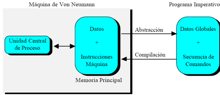
Modelo imperativo (de Labra 1998)
